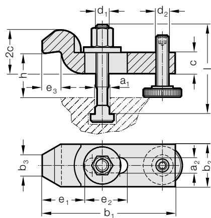
2140.11. Brida acodada, con tornillo de ajuste
